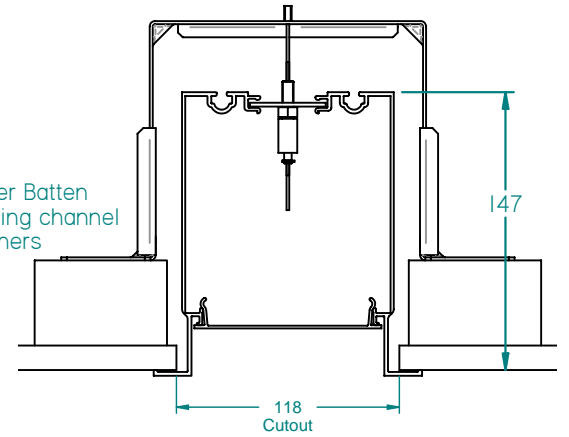
110RB (170RB body)
